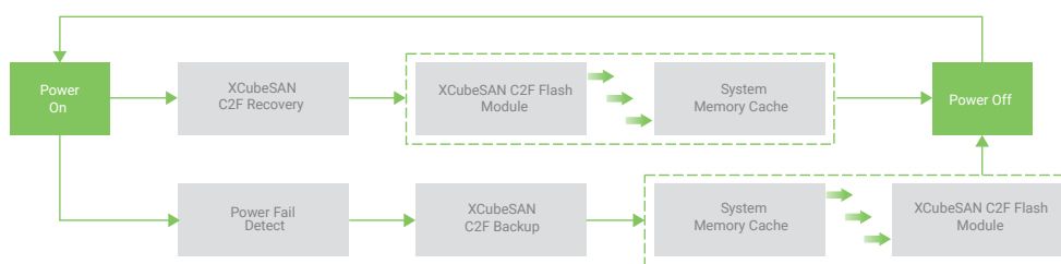
Механизм Cache-to-Flash
